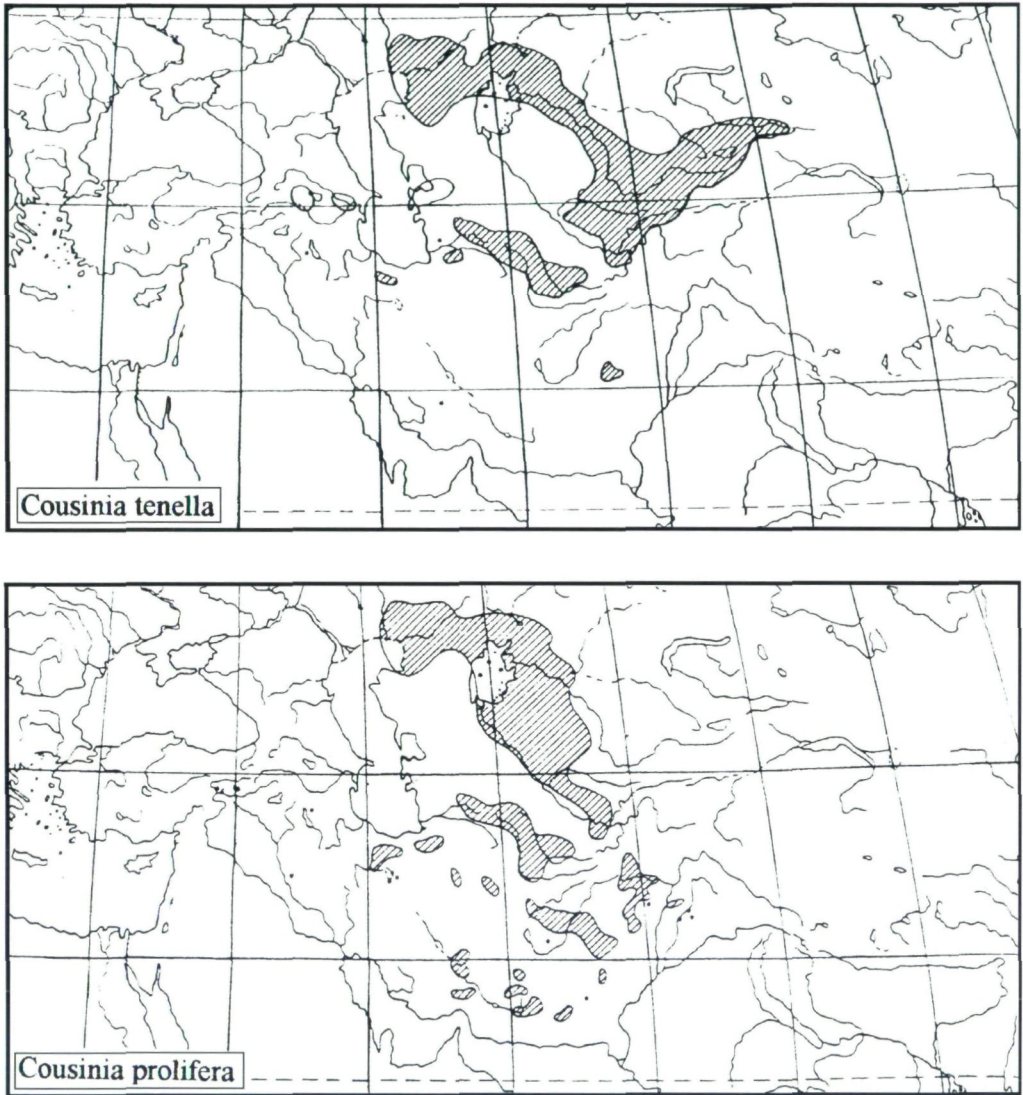
Abb. 3: Gesamtverbreitung von Cousinia prolifera und C. tenella - annuelle Arten mit ausgedehnten Vorkommen in Gebirgsvorländern und in die Niederungen reichenden Arealen (nach KNAPP 1987).
