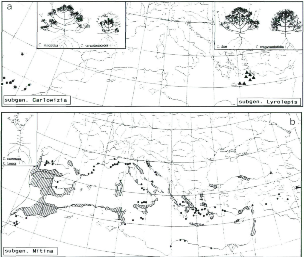
Abb. 1: Verbreitung und Wuchsformschemata der Untergattungen von Carlina (nach MEUSEL & KÄSTNER 1994). Die Arealldifferenzierung entspricht (a) einer Erhaltung ursprünglicher Sippen in zwei Reliktzentren, (b, c) der Ausbreitung von Füllsippen in den zirkummediterranen Raum, und (d, e) dem Vorrücken in die submediterranen Gebirge und nach Mitteleuropa. Als jüngstes Glied ist die wahrscheinlich im Pleistozän ausgegliederte C. biebersteinii (e) zu betrachten, mit der die mediterran-mitteleuropäische Gattung östlich bis zum Baikal vordringt.
