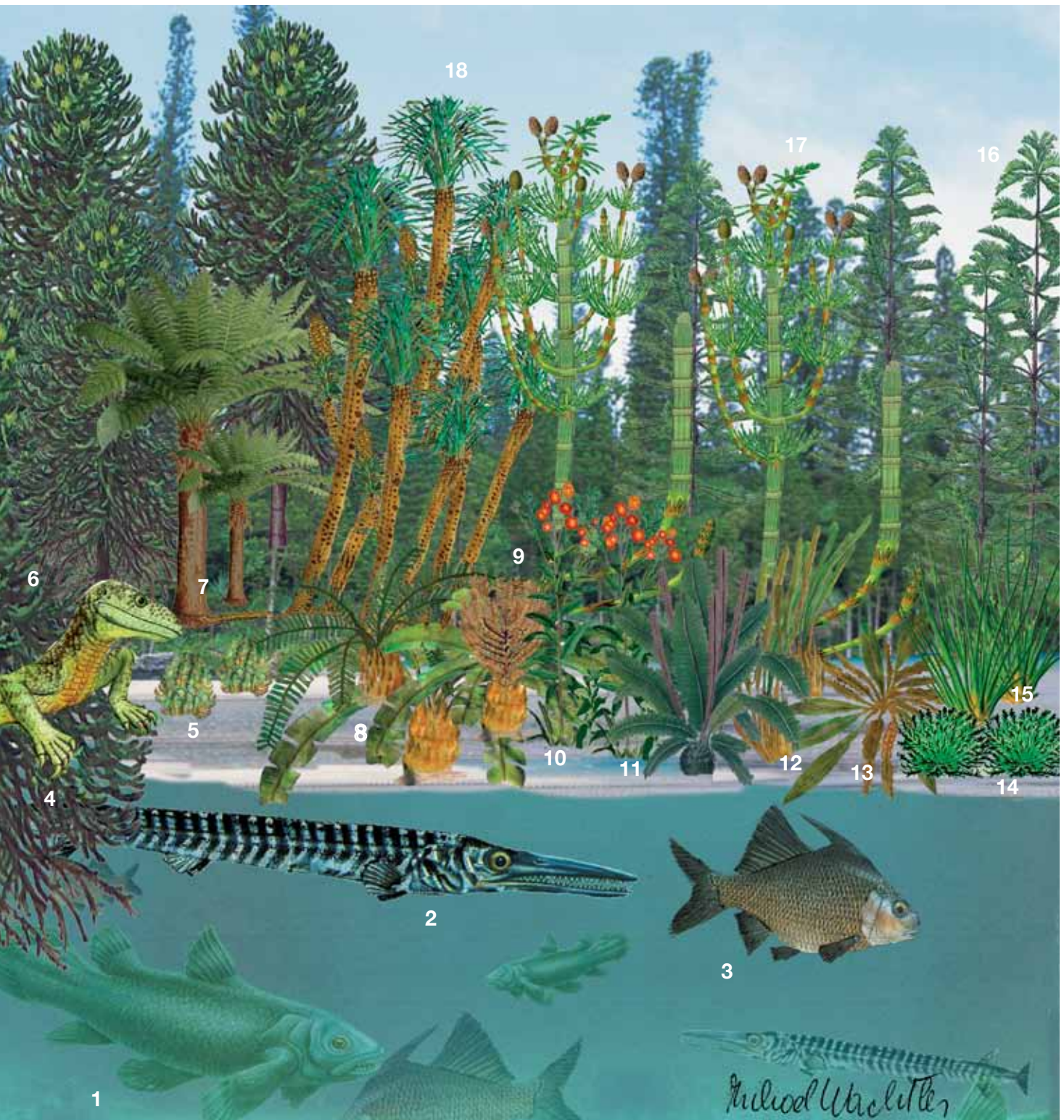
The Anisian landscape from Kühwiesenkopf in the Dolomites (241 million years ago). Reconstruction based on the findings of Michael Wachtler 1999–2009: 1) Coelacanth ; 2) Saurichtys ; 3) Dipteronotus ; 4) Megachirella wachtleri (reptile); 5) Lepacyclotes bechstaedtii (lycopod); 6) Voltzia agordica (conifer); 7) Gordonopteris lorigae (fern); 8) Bjuvia olangensis (cycad); 9) Scytophyllum bergeri (seed fern); 10) Bjuvia olangensis and Dioonitocarpidium cycadea (cycad); 11) Neuropteridium elegans (fern); 12) Pizperesia (cycad); 13) Ladinia simplex (cycad); 14) Selaginellites leonardii (lycopod); 15) Isoetites brandneri (lycopod); 16) Alpia anisica (conifer); 17) Equisetites mougeotii (horsetail); 18) Lycopia dezanchei (lycopod).
