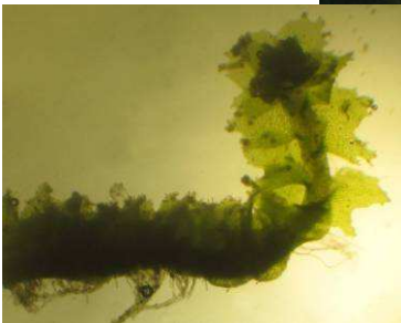
Isopaches bicrenatus
