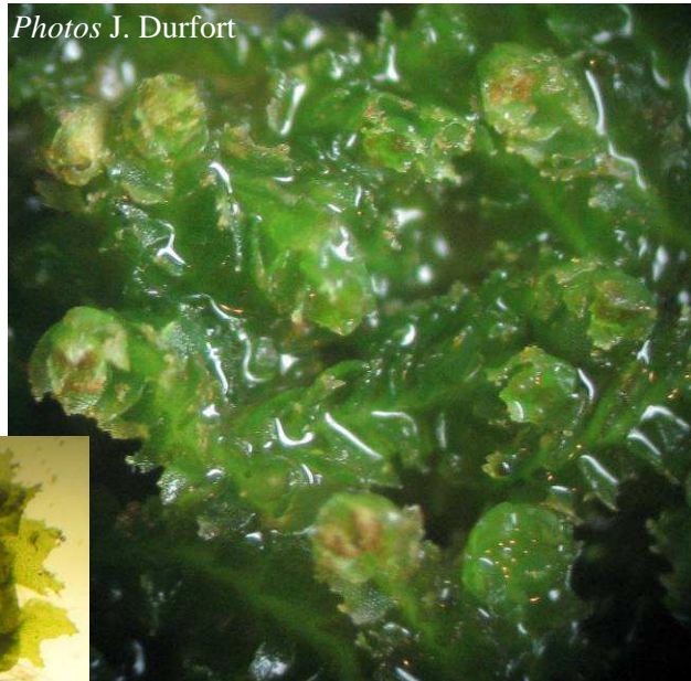
Isopaches bicrenatus
