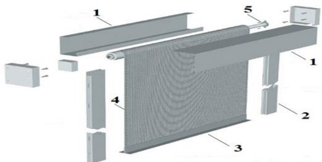
Рис-1. Типовая конструкция автоматических противопожарных штор.
