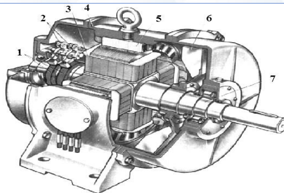
1 -rasm. Sinxron generatori tuzilishi:
