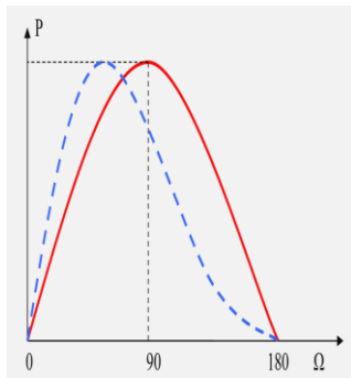
7-rasm. Sinxron generatorni burchak tavsifi. Punktir-ayon qutbli, uzluksiz-noayon qutbli.
