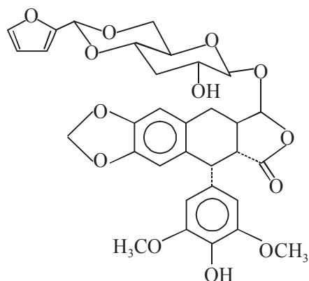
Teniposide
