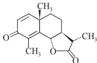
\alpha -Santonin
