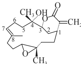
Sinularin
