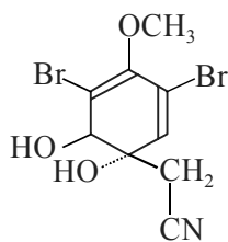
Aerophysinin-1 (+)
