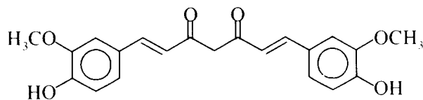
Curcumin
