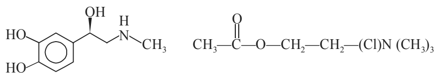
Adrenaline
