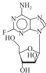
Fludarabine
