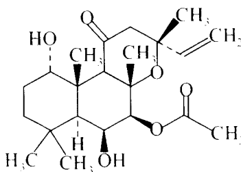
Forskolin [or Colforsin]
