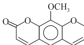
Methoxsalen
