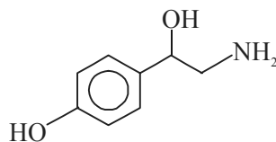
Octopamine
