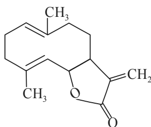
Germacranolide
