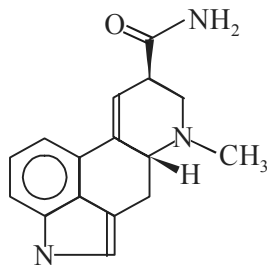
Ergine
