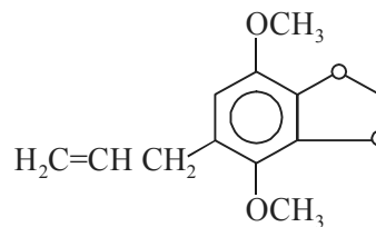
Apiole (Parsley)
