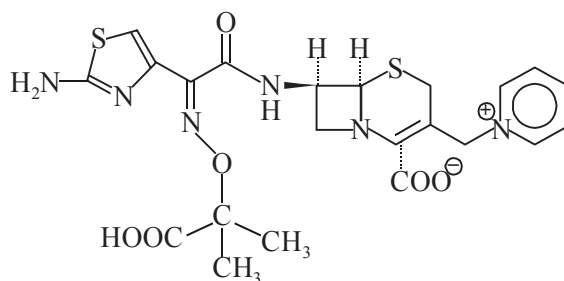
Ceftazidime
