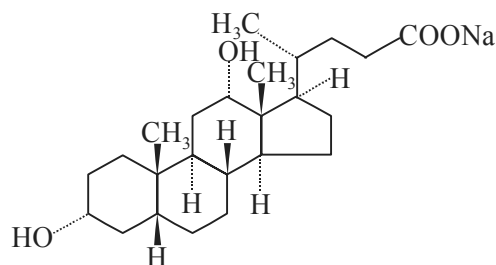
Sodium Desoxycholate
