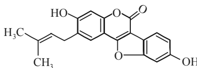
Psolaridin
