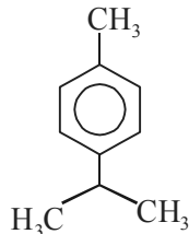
p -Cymene (Dolcymene)
