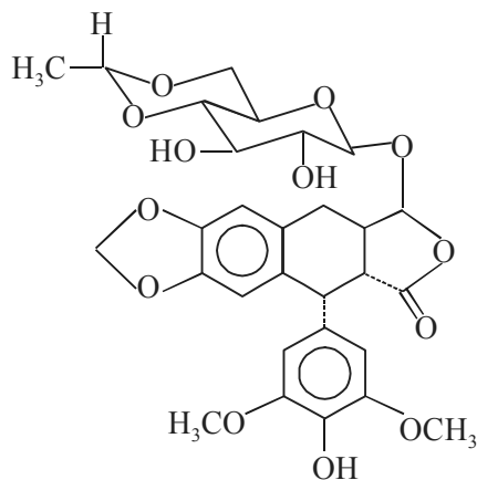
Etoposide
