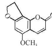
Isobergapten
