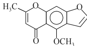
Visnagin
