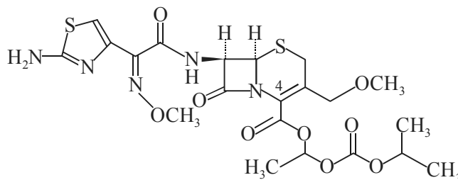
Cefpodoxime Proxetil
