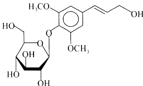
Syringin
