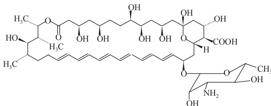
Amphotericin B
