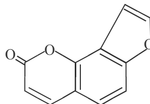
Isopsoralen
