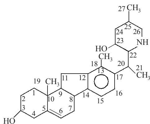
Veratramine [Jeveratrum Alkaloid]
