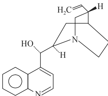
Cinchonine
