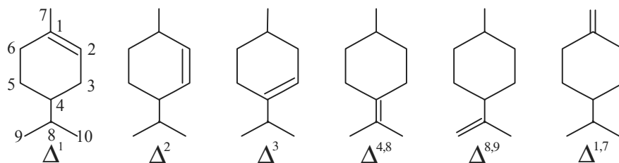
para -Menthenes
