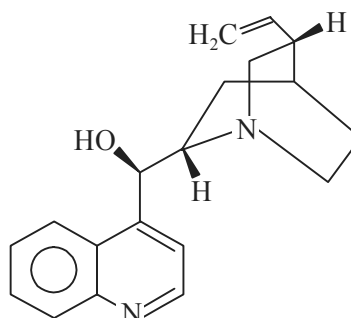
Cinchonidine
