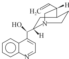
Cinchonidine
