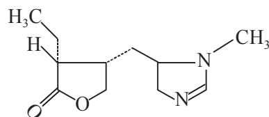
Isopilocarpine
