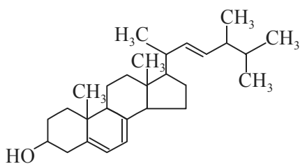
Ergosterol (XIII)
