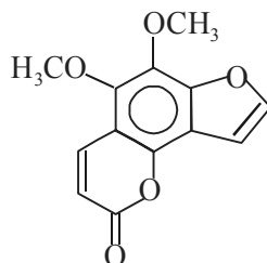
Pimpinellin
