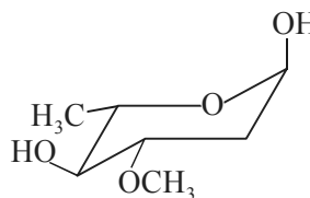
L-Oleandrose
