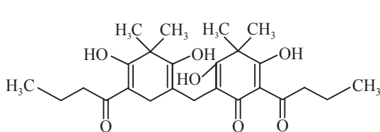
Albaspidin
