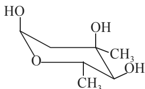
L-Mycarose
