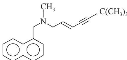
Terbinafine
