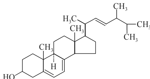
Ergosterol
