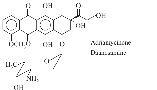
Doxorubicin
