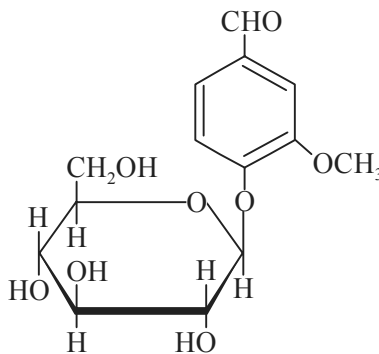
Glucovanillin (Avenein)
