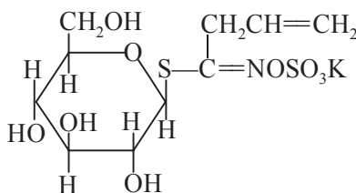
Sinigrin
