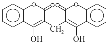
Dicoumarol
