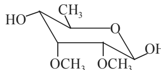
D-Mycinose
