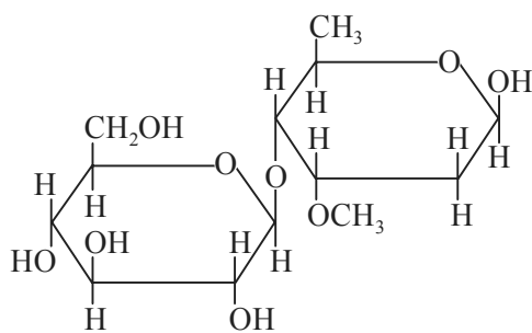
Strophanthobiase
