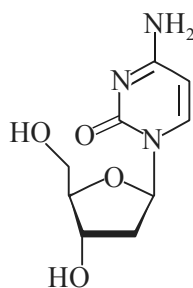
Cytarabine
