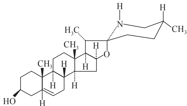
Solasodine
