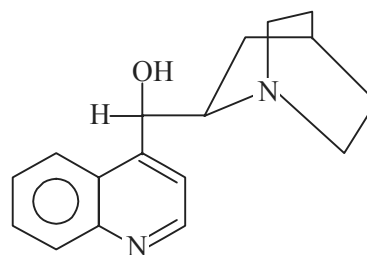
9'-Rubanol
