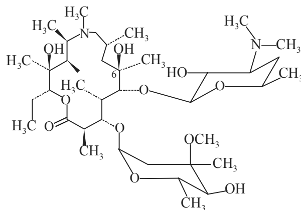
Azithromycin
