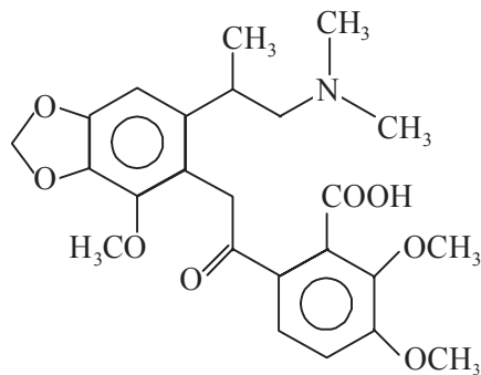
Narceine
