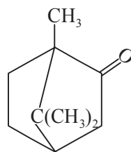
Camphor
