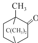
Camphor
