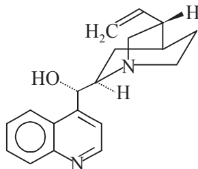
Cinchonine
