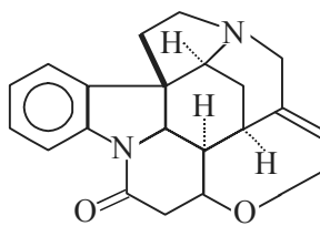
Strychnine
