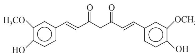
Curcumin
