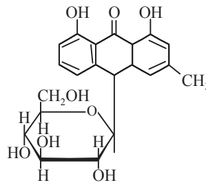
Deoxybarbaloin (Chrysaloin)
