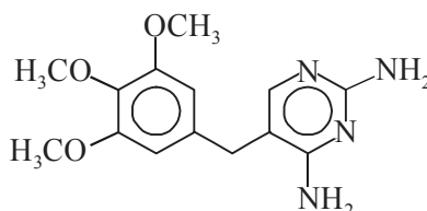
Trimethoprim
