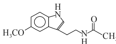
Melatonin
