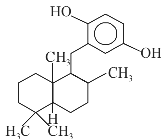
Zonarol
