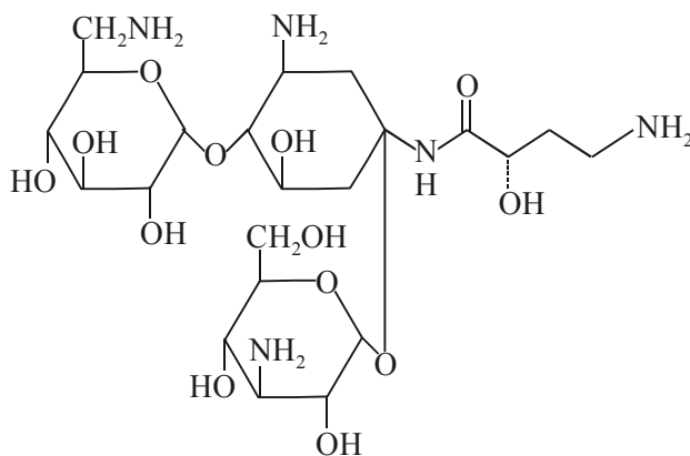
Amikacin
