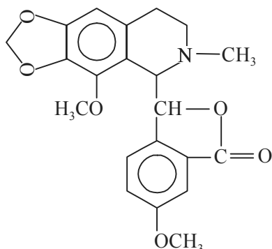
Narcotine
