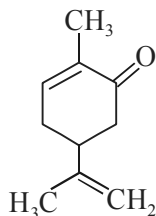
Carvone
