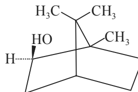
1-Isborneol
