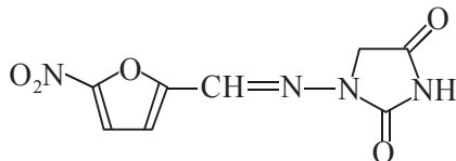
Nitrofurantoin
