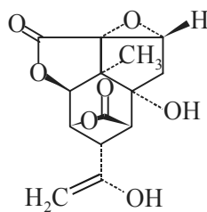
Picrotoxinin
