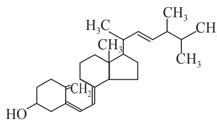
Vitamin D
