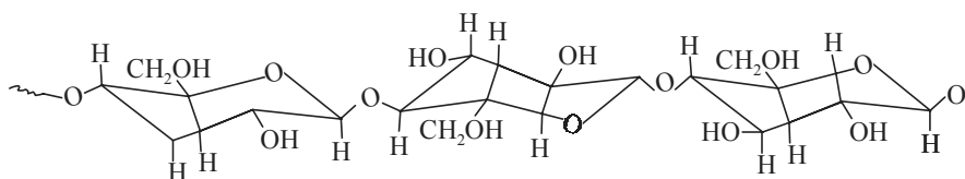
Cellulose
