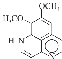
Aaptamine
