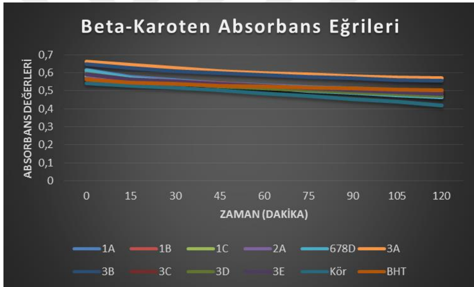
Şekil 28. Ajuga ekstrelerinin \beta -karoten-linoleik asit sisteminde absorban eğrileri
