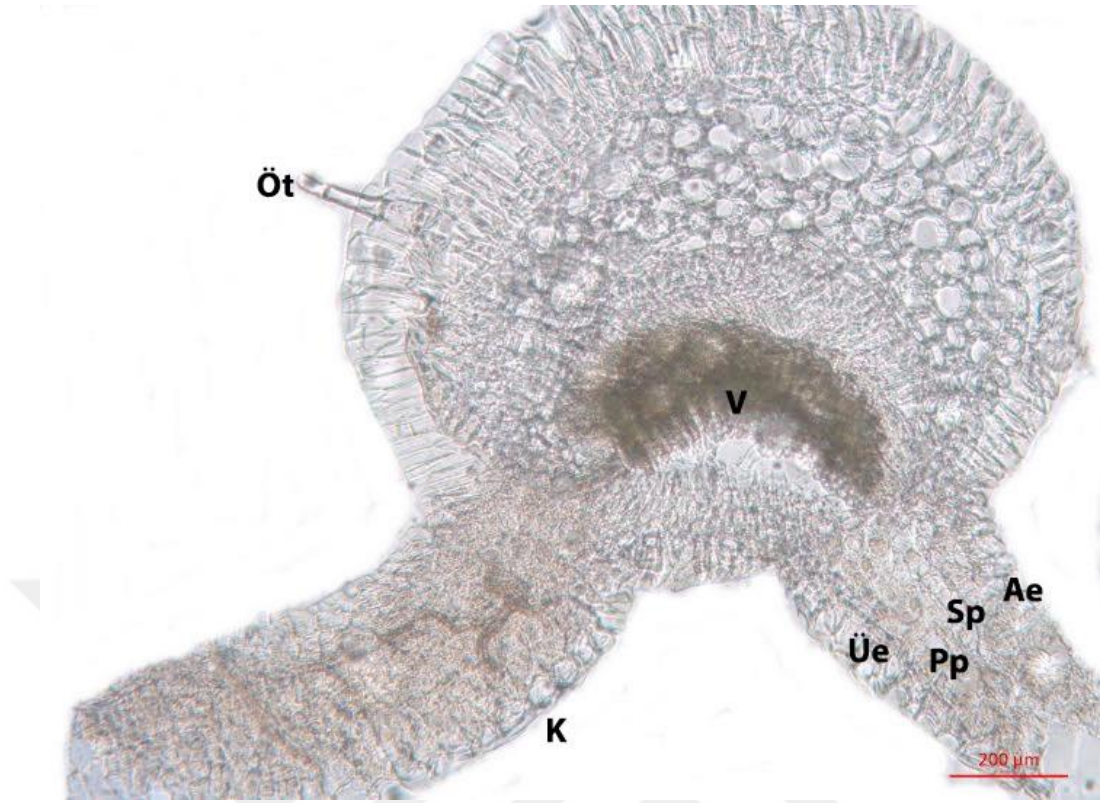
Şekil. 8. A. postii yaprak enine kesiti, Öt: Örtü tüyü, K: Kutikula, Üe: Üst epidermis, Pp: Palizat parenkiması, Sp: Sünger parenkiması, Ae: Alt epidermis, V: Vaskular sistem
