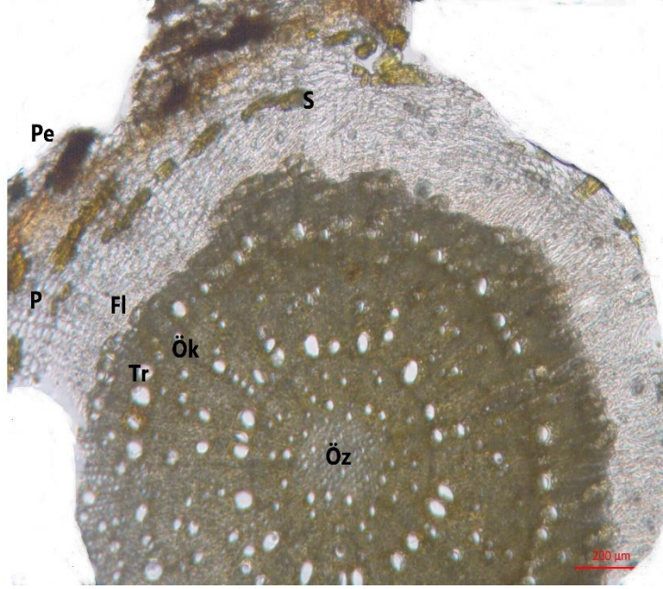
Şekil 11. A. relictta kök enine kesiti, Pe: Periderm, P: Parenkima hücresi, S: Sklerankima, Fl: Floem, Tr: Trake hücresi, Öz: Öz
