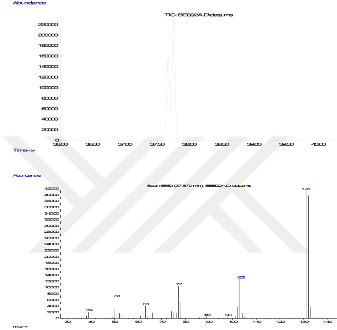
Şekil 30. A. postii uçucu yağ analizi spektrofotometre sonuçları
