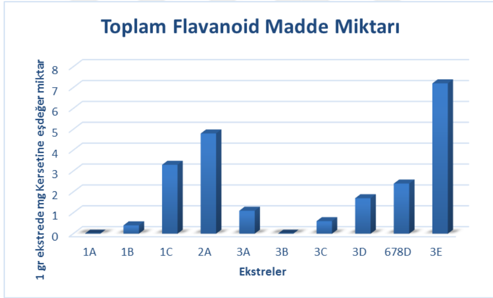
Şekil 18. Ajuga ekstrlerinin toplam flavanoid madde miktarları
