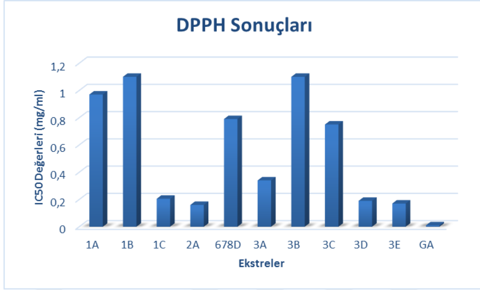
Şekil 25. Ajuga ekstralarının serbest radikal süpürücü etkileri
