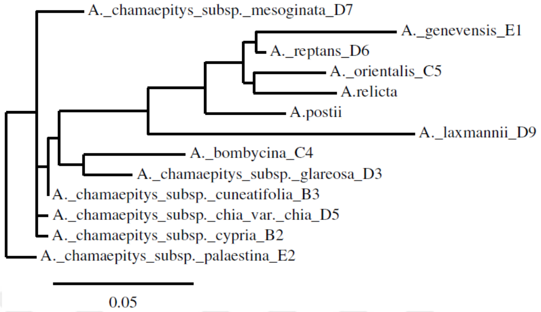
Şekil 32. Bazı Ajuga taksonlarının ITS bölgelerinin baz dizimlerine göre akrabalık ilişkileri
